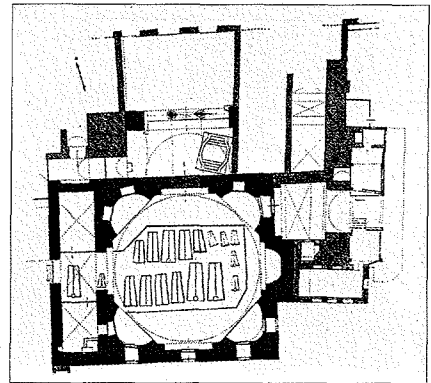
İbrâhim Türbesi'nin planı
